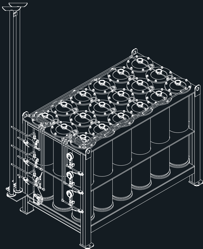
БАГ «Shelf 18.100.3» (Вертикальный)
