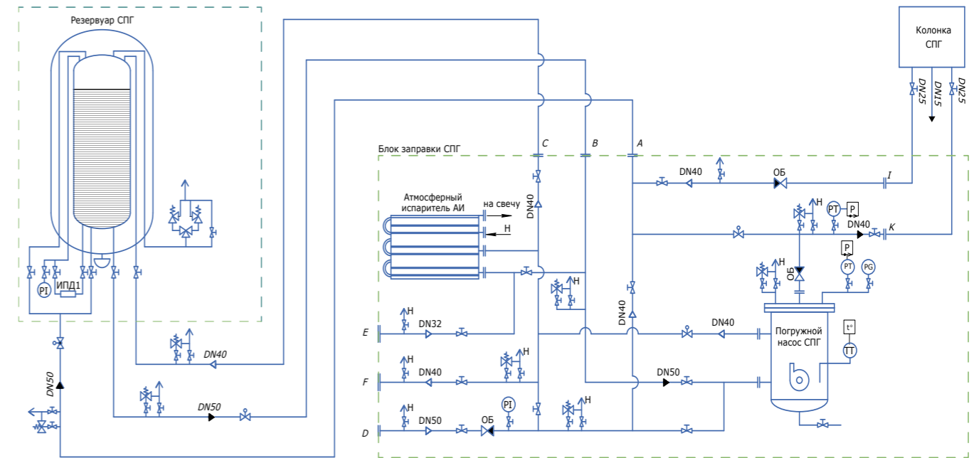
Схема заправочной станции LNG
